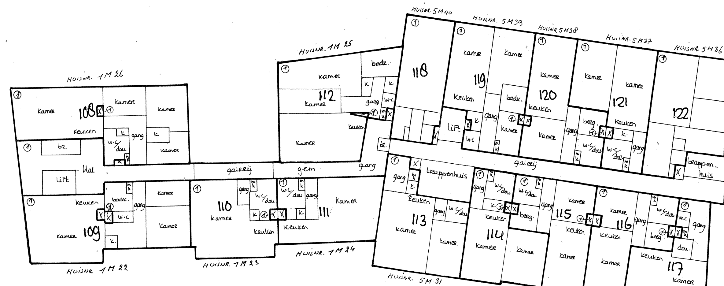
5e verdieping 1:200
