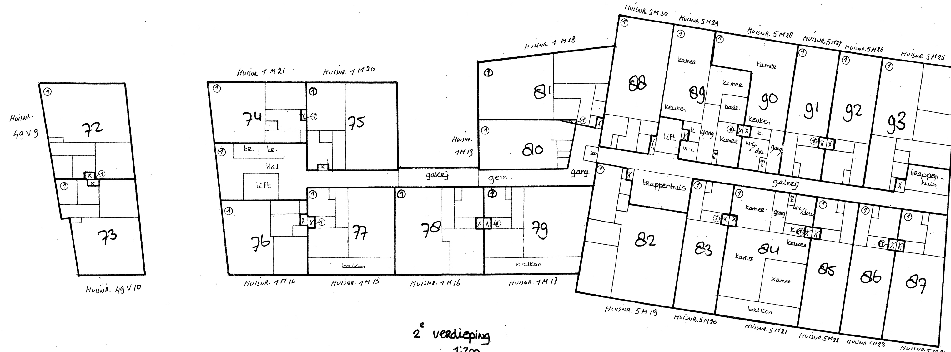
2e verdieping 1:200
